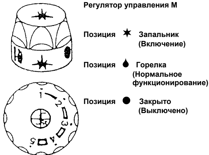
Рис. 4А – Газовый клапан AC3
