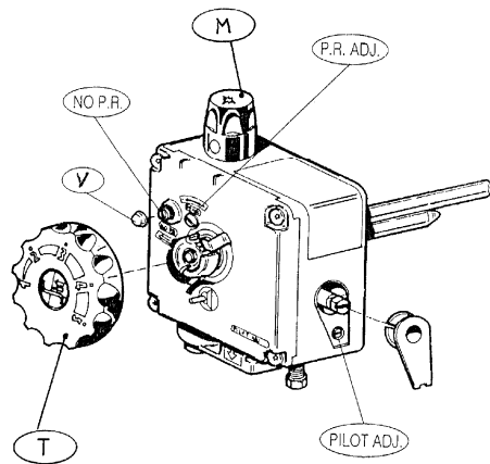
Рис. 4А – Газовый клапан AC3
