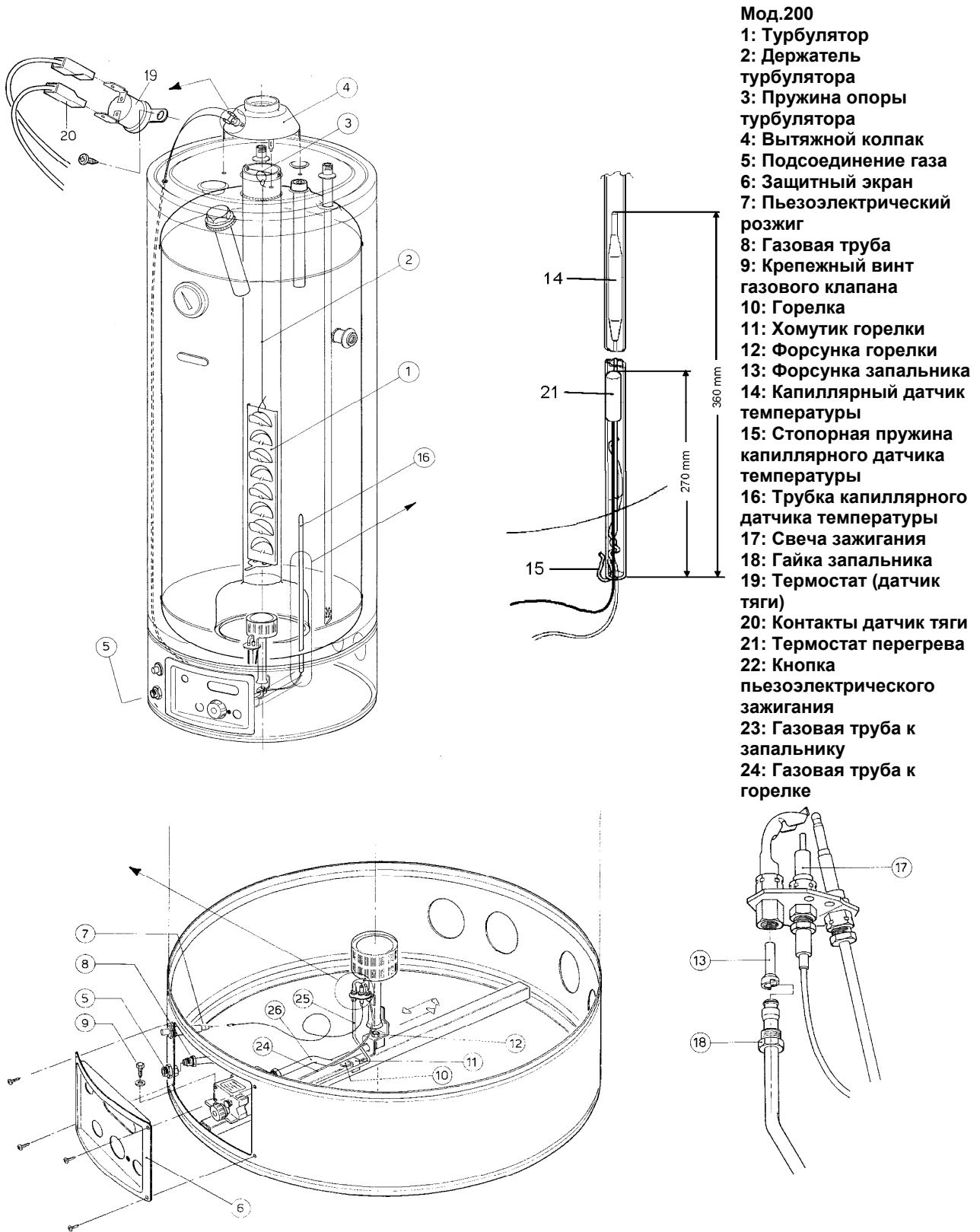
Рис. 2С – ВОДОНАГРЕВАТЕЛЬ НАПОЛЬНЫЙ МОДЕЛЬ 200.
